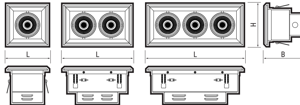
Рис.1 Светильник PSP-S 311
