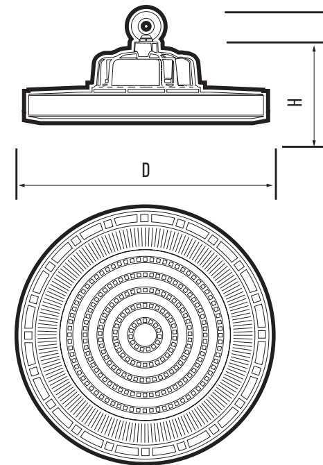
Рис 1. Светильник PHB 05 PRO-5
